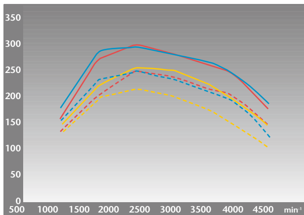
Torque/Nm
