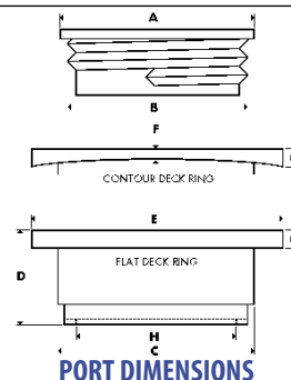
PORT DIMENSIONS
